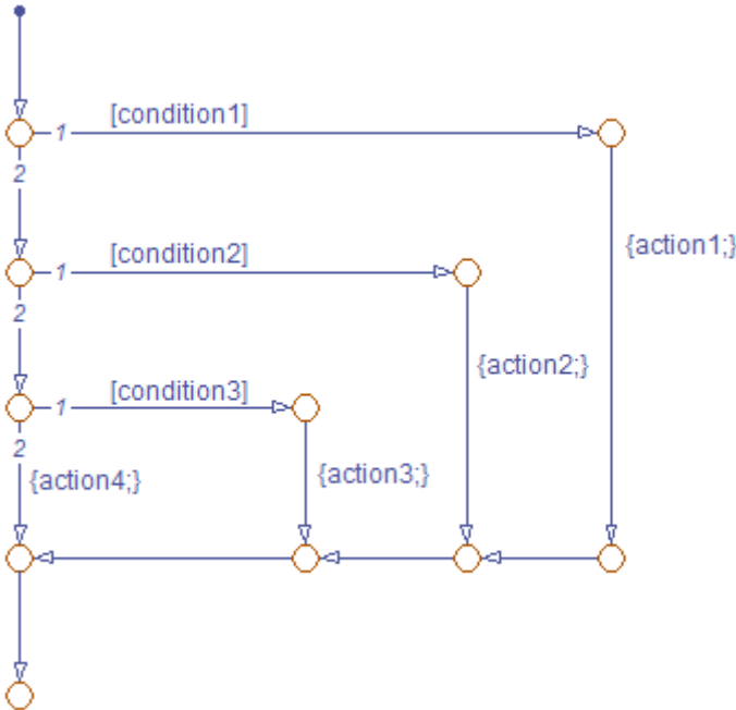
if-elseif-elseif-else
